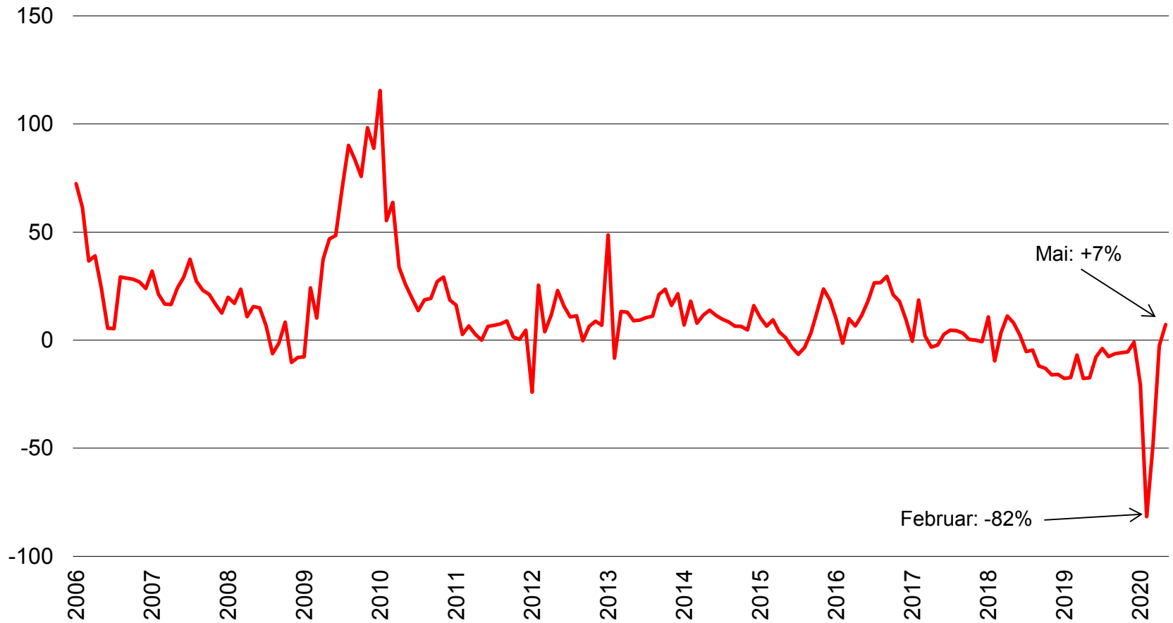
PKW-Verkäufe, in % gegenüber Vorjahr
