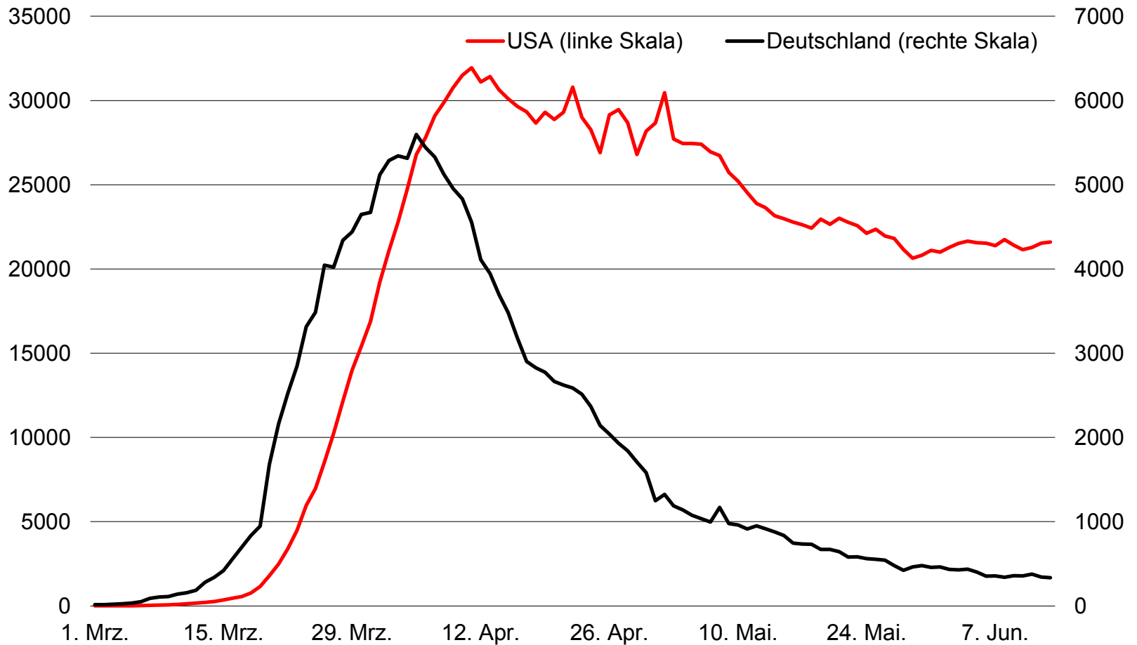
Neue Fälle von COVID-19 (gleitender 7-Tagedurchschnitt)
