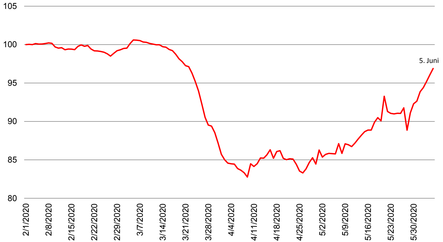
LKW-Maut-Fahrleistungsindex (1. Februar=100; gleitender 7-Tage-Durchschnitt)
